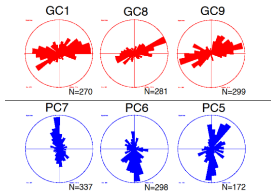
Fig. 1 磁化率異方性における最大軸 (K1) の偏角：地理座標系
