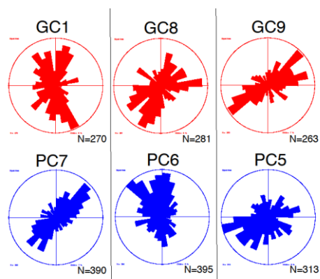
Fig. 2 磁化率異方性における最大軸 (K1) の偏角：サンプル座標系
